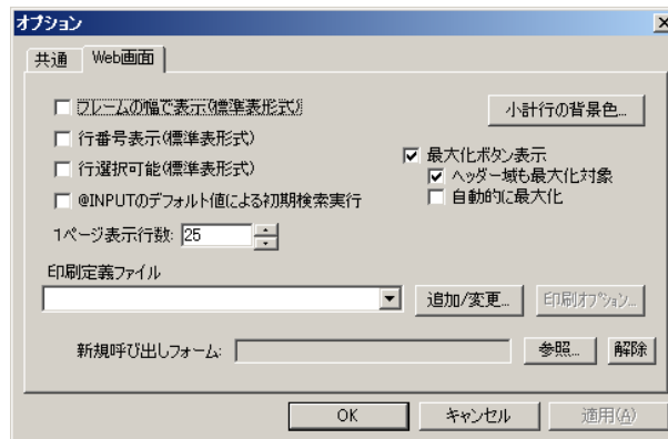
オプション画面 (Web画面タブ)
