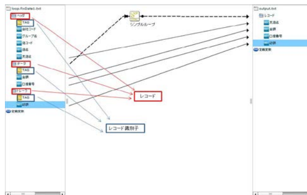
固定長ファイル転送におけるループ処理
