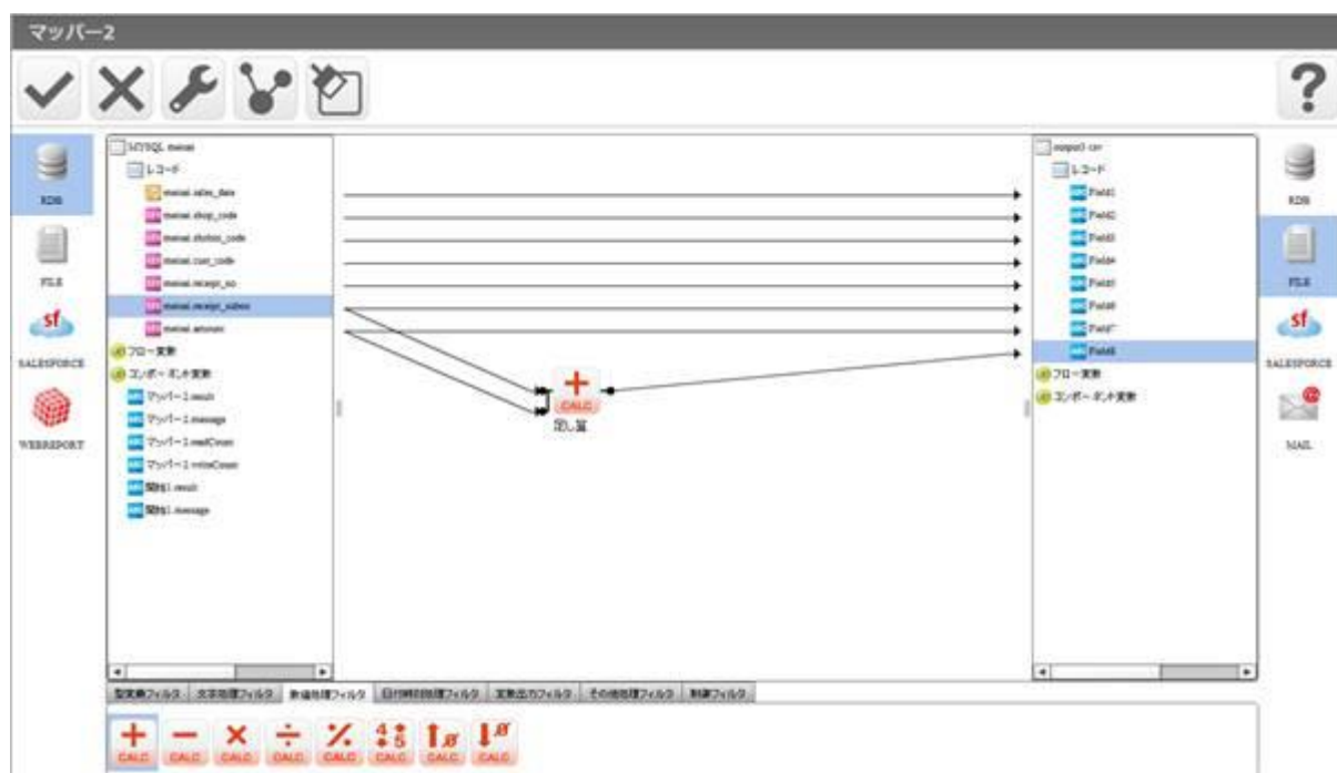
Mapper編集画面（アイコン拡大サイズ表示）
