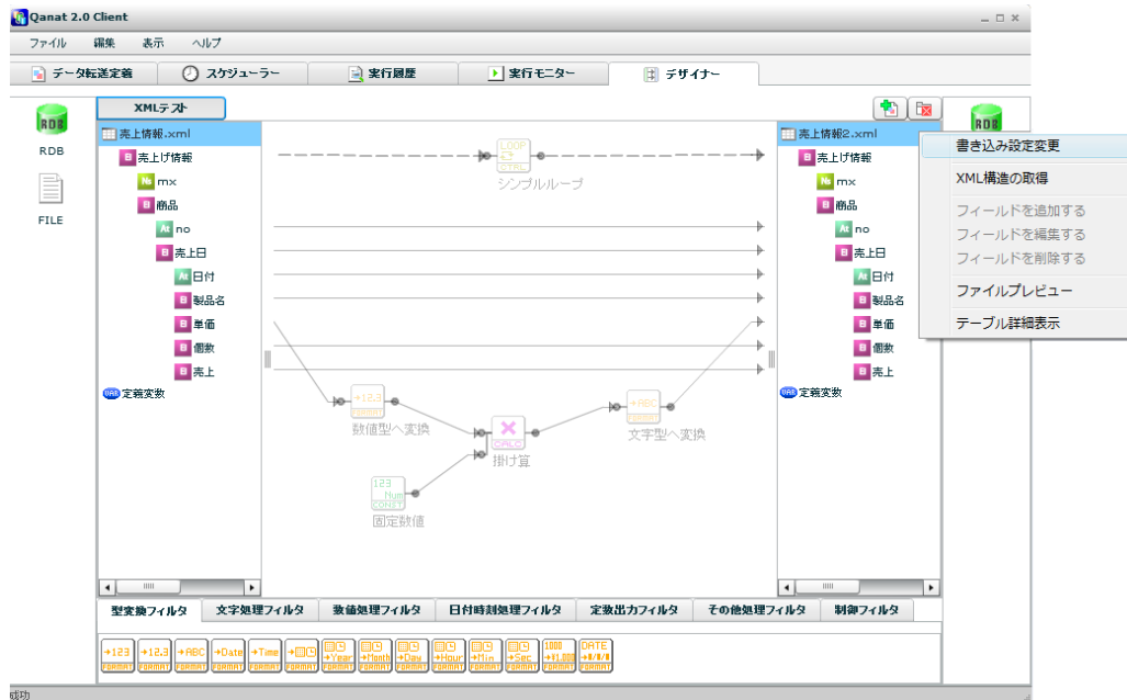
転送先 XML ファイルを右クリックで表示されるメニュー
