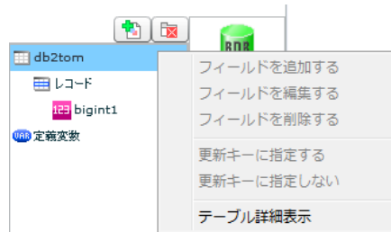
転送先テーブルを選択時に右クリックで表示されるメニュー
