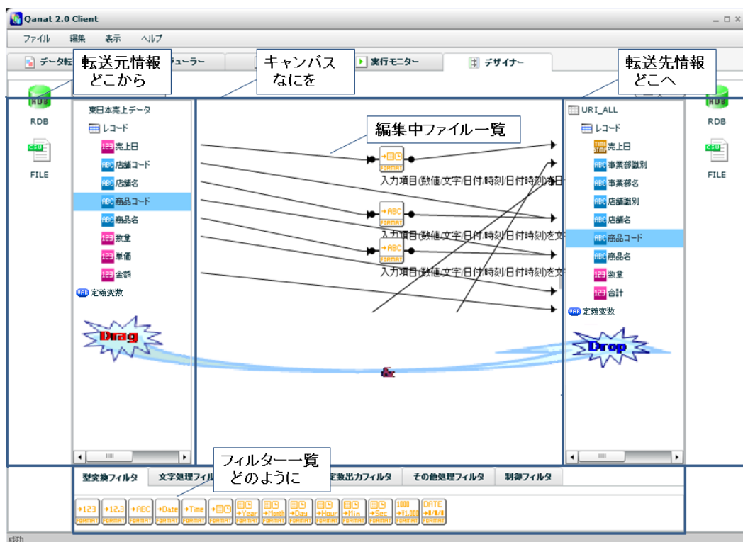
デザイナー画面
