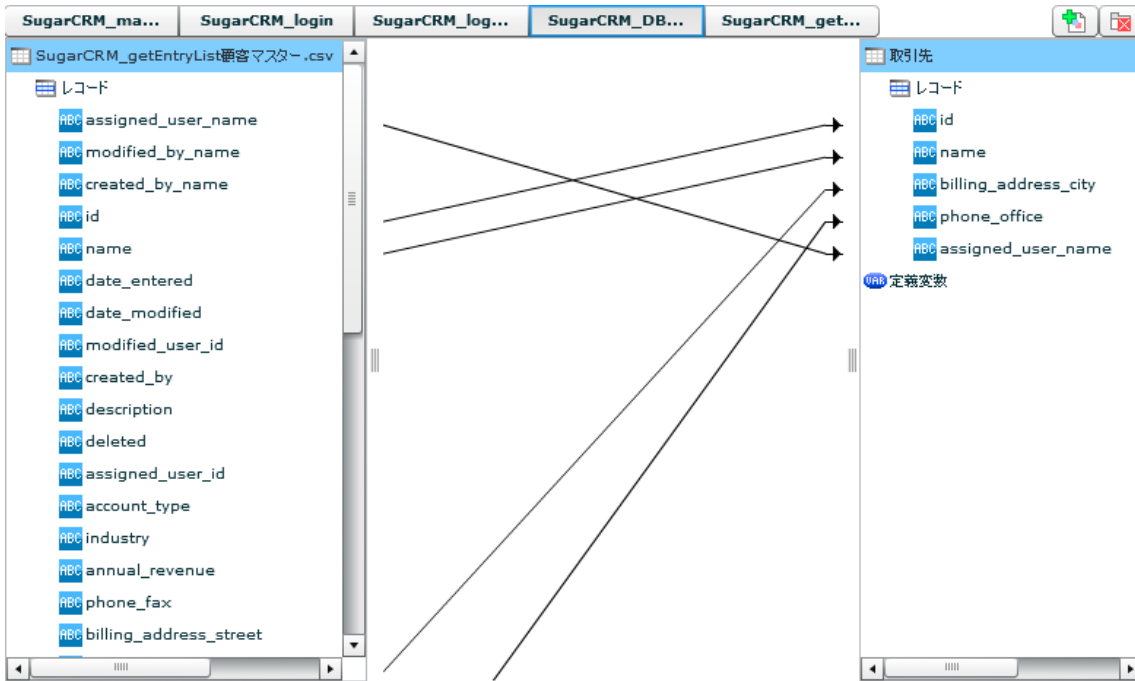
SugarCRM_DB2UPDATE 定義
